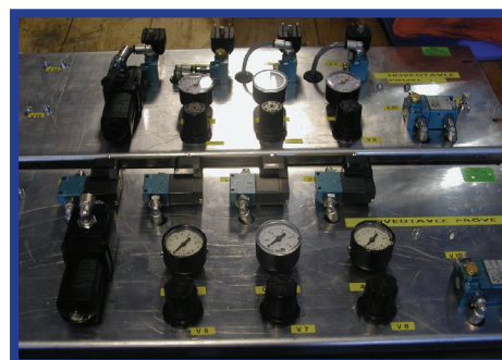
Контрольная панель
